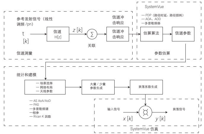
图 3. MIMO 信道测量、参数提取、建模和仿真
